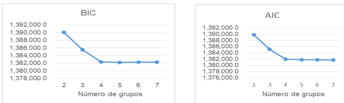
Gráfica 1. Criterios de información BIC y AIC
